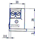
Západka zavřená.
