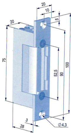
Západka otevřená.
